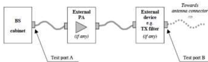
Gambar 3. Test port dari Transmitter .
