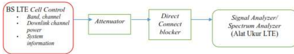
Gambar 5. Bagan Pengujian Perangkat BS LTE FDD-TDD.
