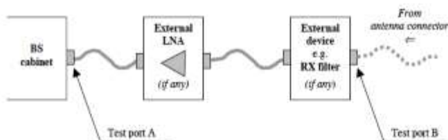
Gambar 4. Test Port Penerima.
