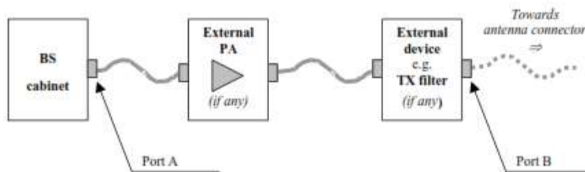
Gambar 1. Interface pemancar BS type 1-C.
