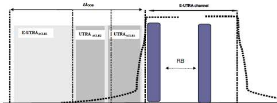
Gambar 3. Persyaratan ACLR
